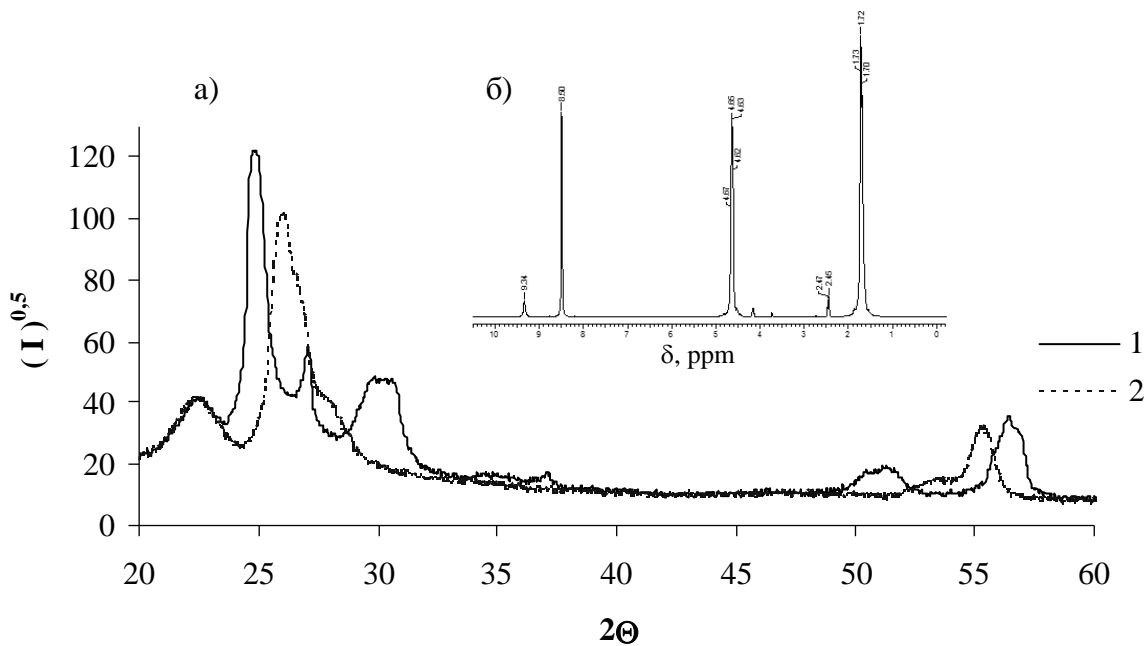
Рис. 1. Дифрактограммы нитрата-ацетата графита (1) и выдержанного затем в этилформате (2) в течение 120 ч (а); ЯМР ^1\text{H} спектр образца этилформиата после обработки нитрата-ацетата графита (б)
