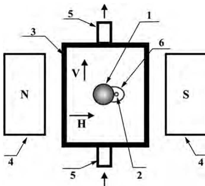
Рис. 1. Схема установки для исследования эффективности улавливания имплантата
