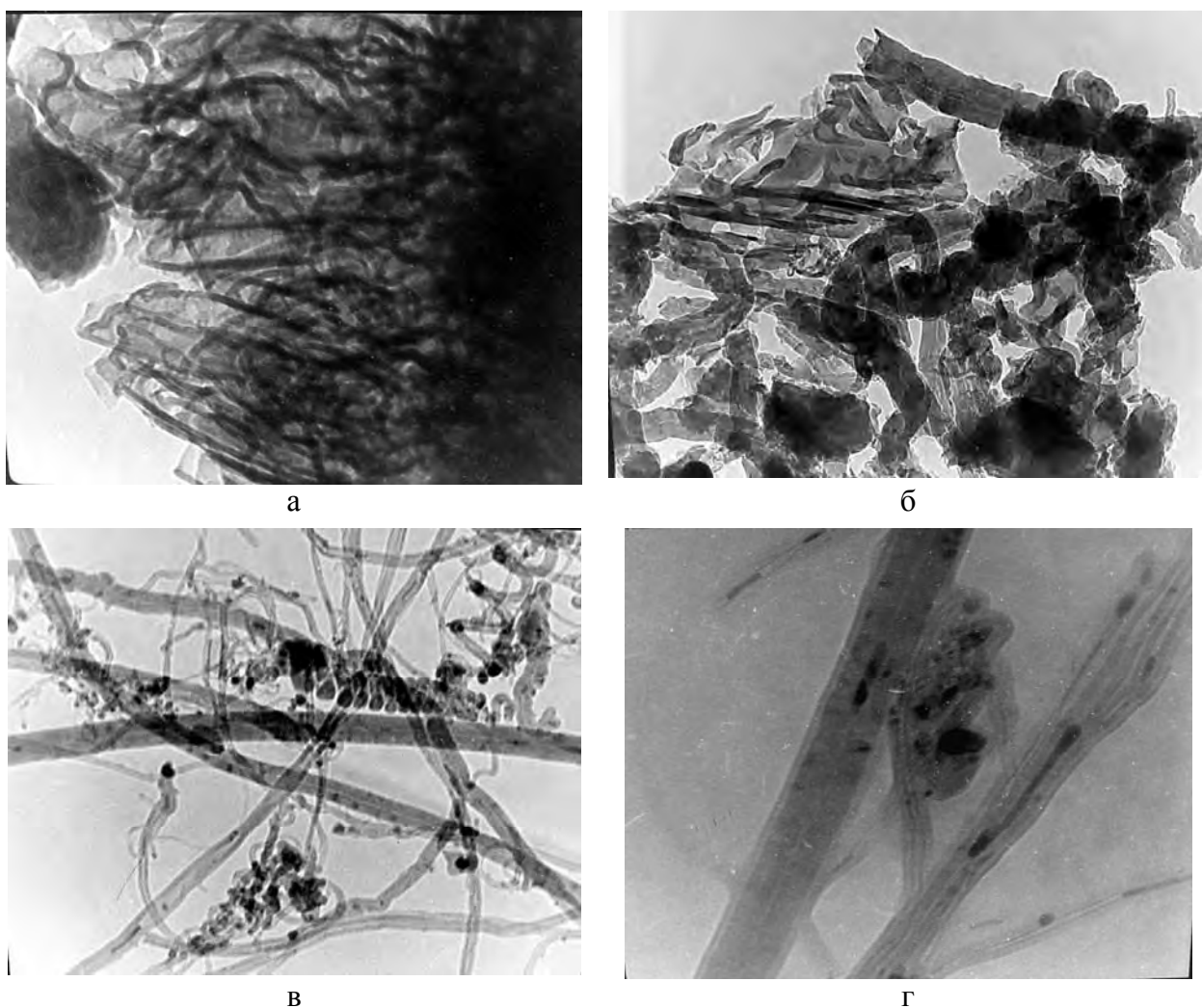
Рис. 2. ТЭМ изображение: а) углеродный продукт (Pr-But, Fe/ \text{CaCO}_3 , He, 800°C); б) углеродный продукт (Pr-But, He, Fe/ \text{CaCO}_3 , 800°C); в) углеродный продукт (Pr-But, He, ферроцен, 800°C); г) углеродный продукт (Pr-But, He, ферроцен, 800°C)
