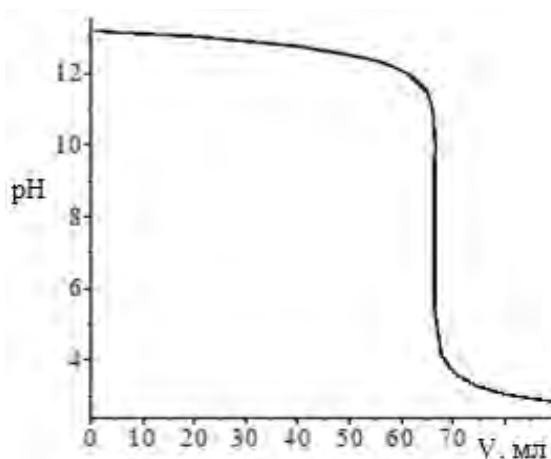
Рис. 2. Кривая кислотно-основного титрования 0,1 М Ва(ОН) 2 раствором 0,1 М Н 3 Р 4
