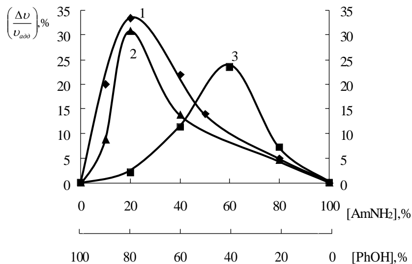
Рис. Зависимость критерия \left(\frac{\Delta v}{v_{add}}\right) от состава смеси кверцетина (PhOH)
