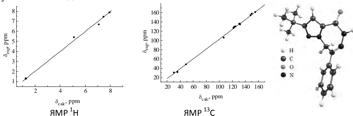
Рис. Равновесная конфигурация и линейные корреляции между экспериментальными и рассчитанными методом GIAO химическими сдвигами ядер ^1\text{H} и ^{13}\text{C} 2- трет -бутил-7-фенил-5,8-дигидро-4 H -пиразоло[5,1- d ]-[1,2,5]триазепин-4-она
