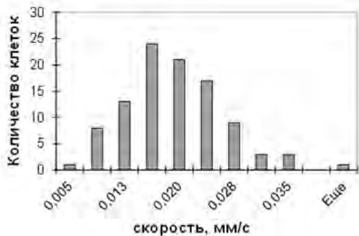
Рис. 1. Гистограмма распределения ФЭЧ по магнитофоретическим скоростям для времени инкубации t_i=4 суток
