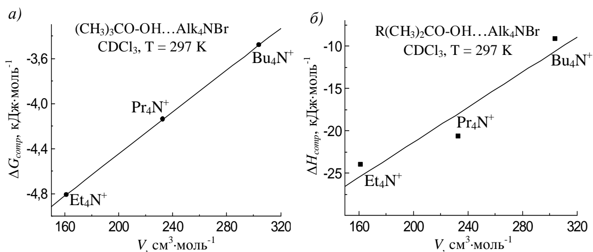
Рис. 2. Зависимости свободной энергии Гиббса образования комплекса (\text{CH}_3)_3\text{CO-OH}\dots\text{Alk}_4\text{NBr} (а) и энтальпии комплексообразования \text{R}(\text{CH}_3)_2\text{CO-OH}\dots\text{Alk}_4\text{NBr} (б) от собственного объема катиона ( V ) \text{Alk}_4\text{NBr} ( \text{CDCl}_3 , T = 297 \text{ K} )
