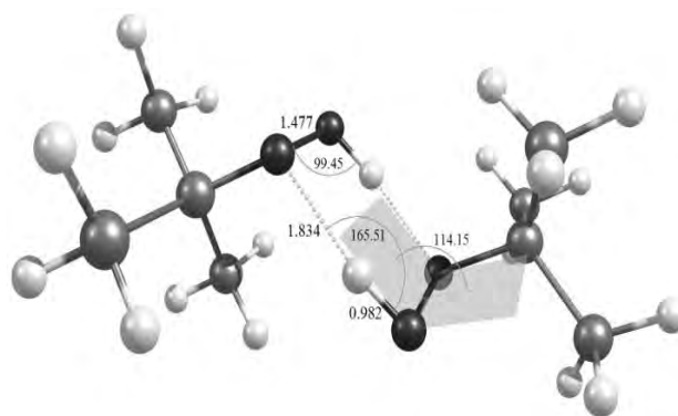
Рис. 3. Структурная модель димера (\text{CH}_3)_3\text{CO}-\text{OH} (оптимизация молекулярной геометрии выполнена в приближении метода \text{MP2}/6-31\text{G}(\text{d},\text{p}) )
