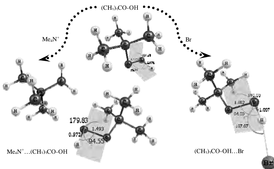
Рис. 4. Равновесные конфигурации гидропероксида трет -бутила и его ассоциатов с ионами \text{Me}_4\text{NBr} (оптимизация молекулярной геометрии выполнена в приближении метода \text{MP2}/6-31\text{G}(\text{d},\text{p}) )
