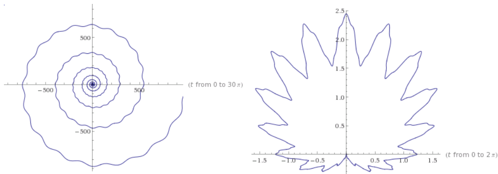
Рисунок 1 – Графики функций
