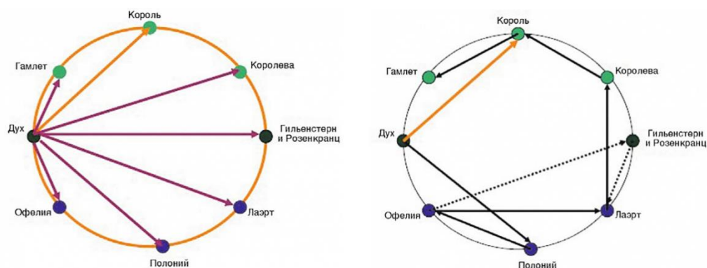
Рис. 1. Анализ пьесы Шекспира «Гамлет» с помощью теории графов: а) граф намерений Духа покойного короля; б) граф цепочки событий
