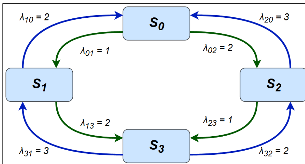
Рисунок 3 – Граф Марковского процесса (составлено по [8])
