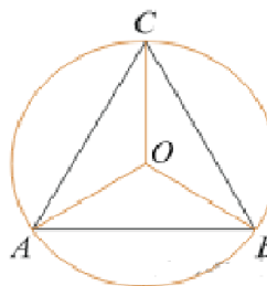
Рисунок 2 – Правильный треугольник, вписанный в окружность
