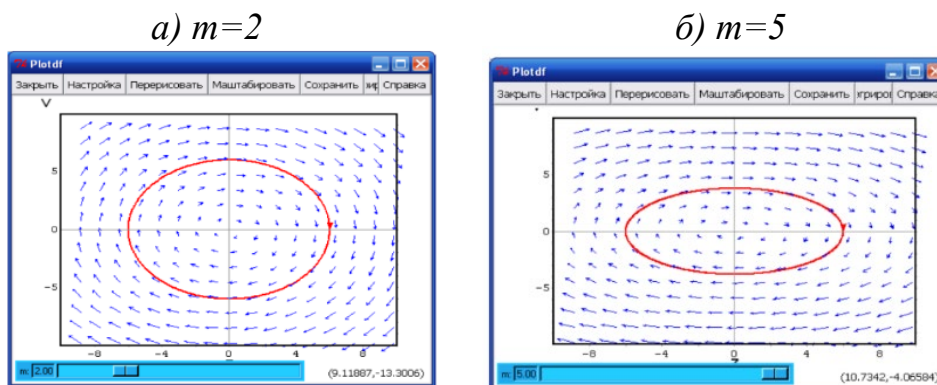
Рисунок 3 – Поле направлений системы дифференциальных уравнений для m=2 а) и m=5 б)
