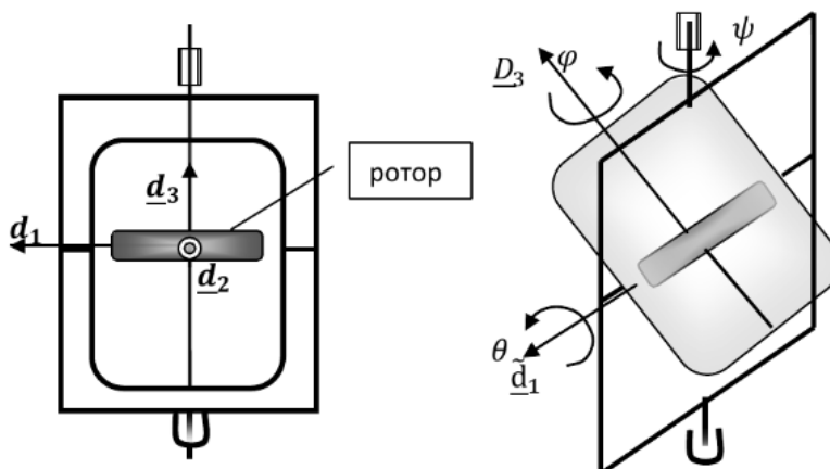
Рисунок 4 – Иллюстрация к задаче 6, слева – статическое состояние ротора, справа – в движении (поворот)
